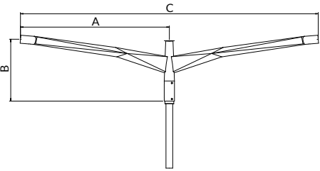
staffa per doppia luce
